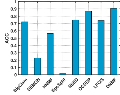
Fig. 3: Node-level analysis.
